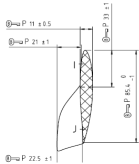
Schnitt / Section A-A
