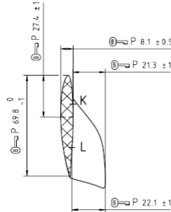
Schnitt / Section B-B
